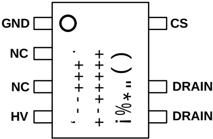
图 2 管脚封装
